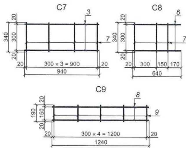
Рисунок Б.11 — Арматурные сетки C7, C8, C9
