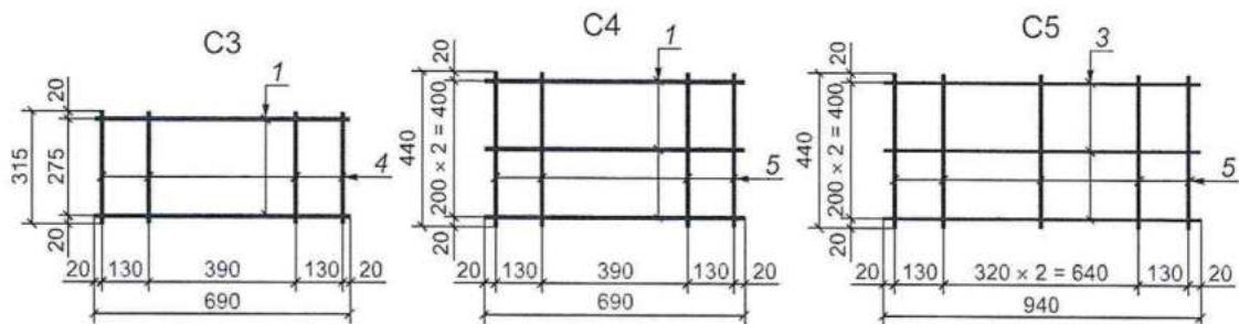
Рисунок Б.9 — Арматурные сетки C3, C4, C5
