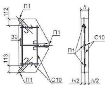
Рисунок Б.6 — Армирование тротуарной плиты 11Д
