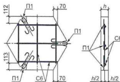
Рисунок Б.4 — Армирование тротуарной плиты 3Ш
