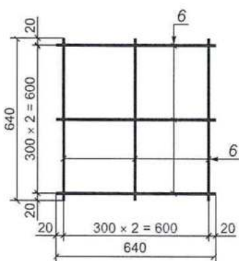
Рисунок Б.10 — Арматурная сетка C6
