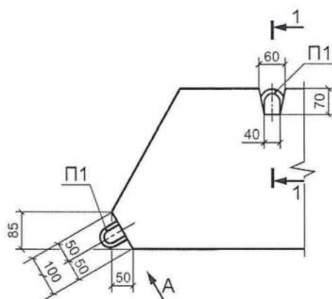
Рисунок Б.1 — Детали установки петель П1
