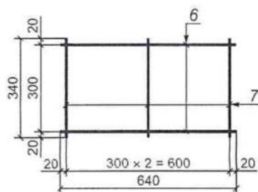
Рисунок Б.12 — Арматурная сетка С10
