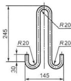
Рисунок Б.13 — Петля П1
